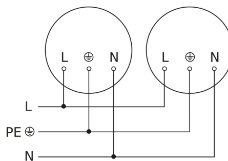
aansluitschema Master/slave koppelin
